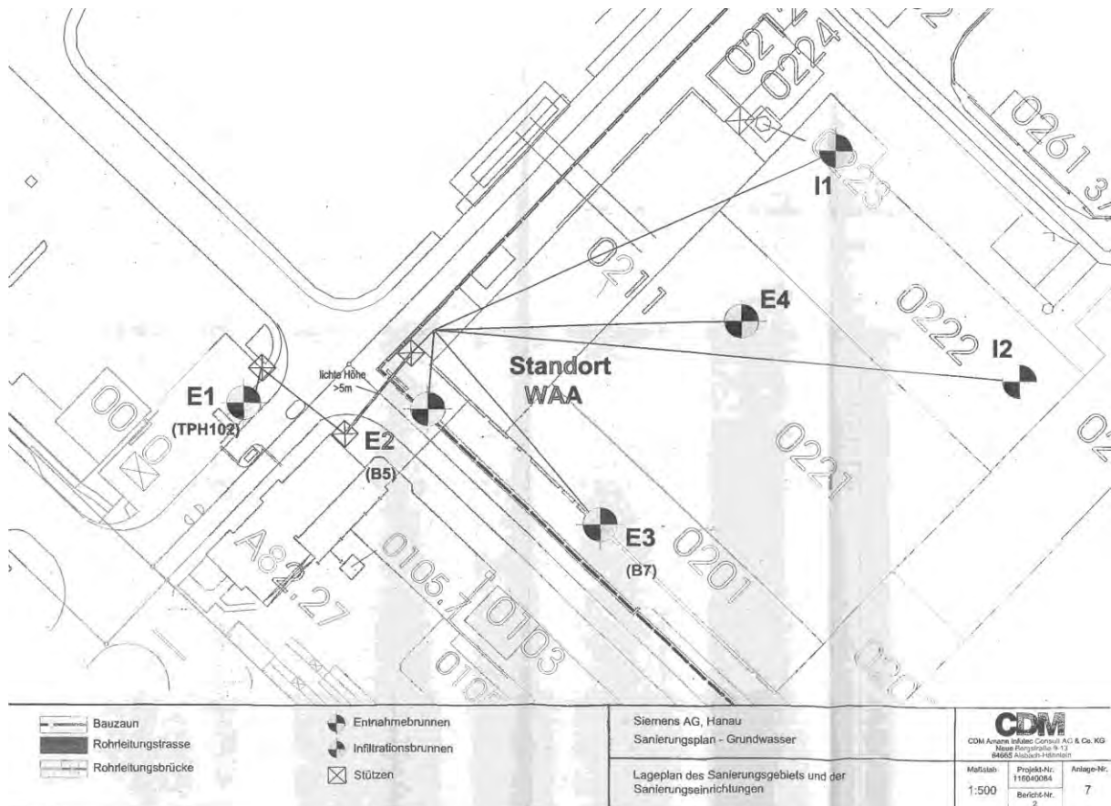
Abbildung 4: Lage der Entnahme- und Infiltrationsbrunnen
